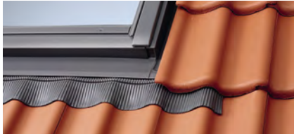
EZ 6000 Ziegel wärmegeklämmt, EZ 1000 Ziegel
