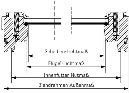
Querschnitt
