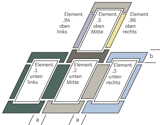
Asymmetrische Kombi-Eindeckrahmen
