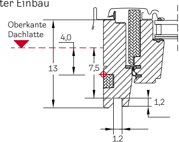
Vertiefter Einbau
